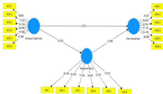
Gambar 2. Hasil Uji Bootstrapping Sumber: Hasil analisa data (2024)
